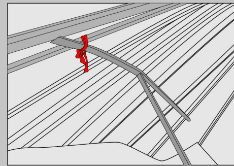
УЗЕЛ 1 подпорка под задние скатные жерди
